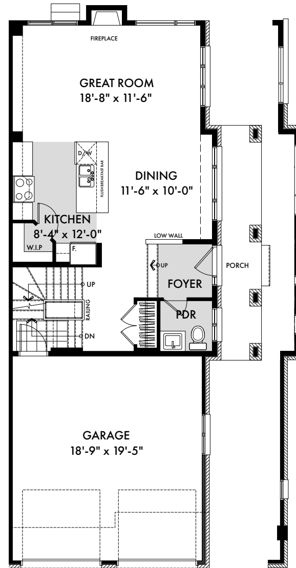
ELEV A
